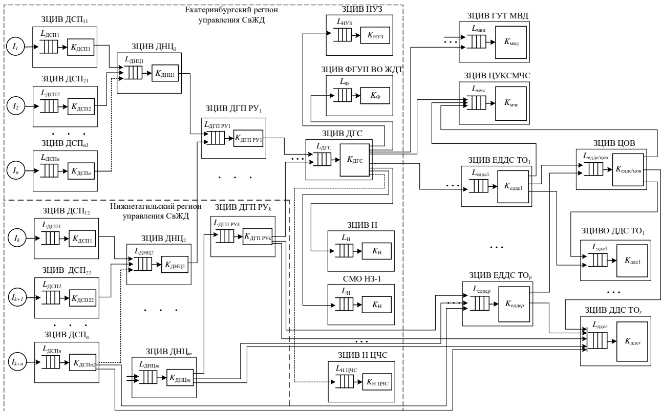
Рисунок 2 – Алгоритмическая модель процесса реагирования при возникновении НиЧС на железной дороге во время перевозочного процесса
