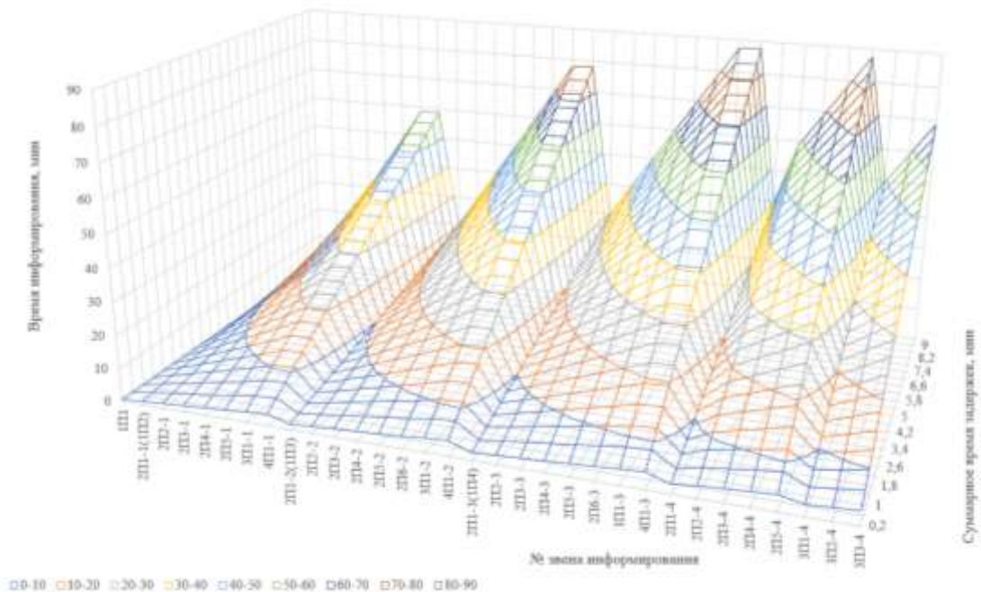
Рисунок 6 – Время передачи информации о возникшей НиЧС в цепях информационного взаимодействия, формируемых звеньями высшего порядка 1П – 4П при изменении суммарного времени задержек на каждом ЗЦИВ
